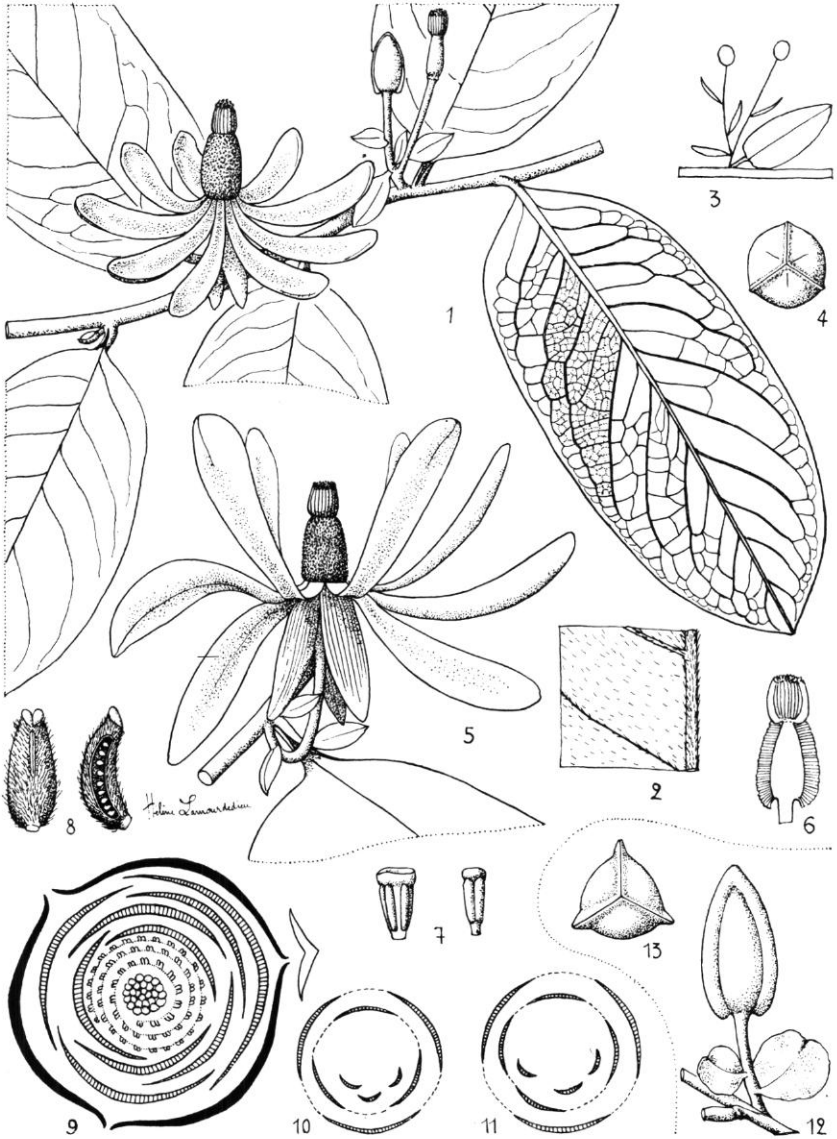
Pl. 1. — Toussaintia Hallei A. Le Thomas : 1 , rameau florifère \times 2/3 ; 2 , détail de la pubescence face inférieure de la feuille \times 2 ; 3 , schéma d'une inflorescence; 4 , bouton, vue apicale \times 1,5 ; 5 , fleur, gr. nat.; 6 , coupe de l'androgynophore \times 1,5 ; 7 , étamines \times 8 ; 8 , carpelle, et coupe \times 4 ; 9 , diagramme floral; 10 , 11 , diagramme montrant le nombre et la position variables des pétales (N. Hallé 4189, d'après un sujet vivant). — T. congolana Boutique : 12 , bouton floral et bractées, gr. nat.; 13 , bouton floral, vue apicale \times 1,5 (Wagemans 1677).
